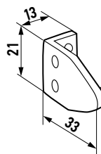
Держатель карниза для нижней фиксации 240175-0000
