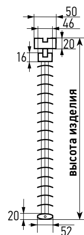
Вид сбоку
