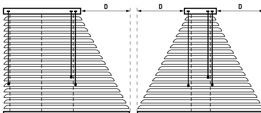
Полутрапеция
