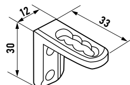
Кронштейн нижний тип В пластмассовый 249181-0000
