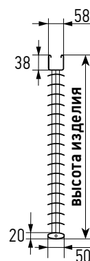
Вид сбоку Алюминий 50 мм
