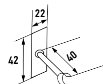
Фиксатор прозрачного прута для крепления к окнам ПВХ 249184-0000
