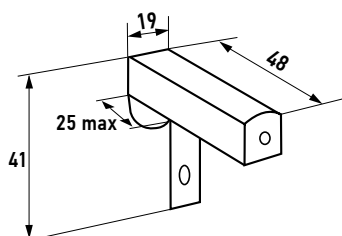
Кронштейн для окон ПВХ верхний 249182-0000
