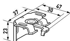
Универсальный кронштейн 240180-0000
