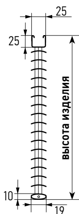
Вид сбоку
