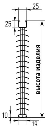
Вид сбоку
