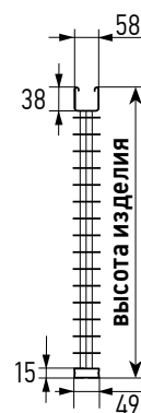
Вид сбоку Пластик 50 мм
