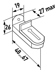
Кронштейн для окон ПВХ нижний 249183-0000
