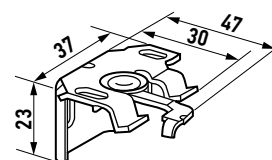
Кронштейн 240180-0000
