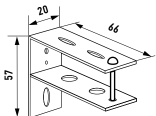
Установочный кронштейн 245780
