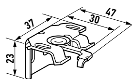
Универсальный кронштейн 240180-0000
