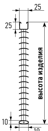
Вид сбоку
